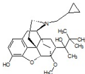
Buprenorphine
